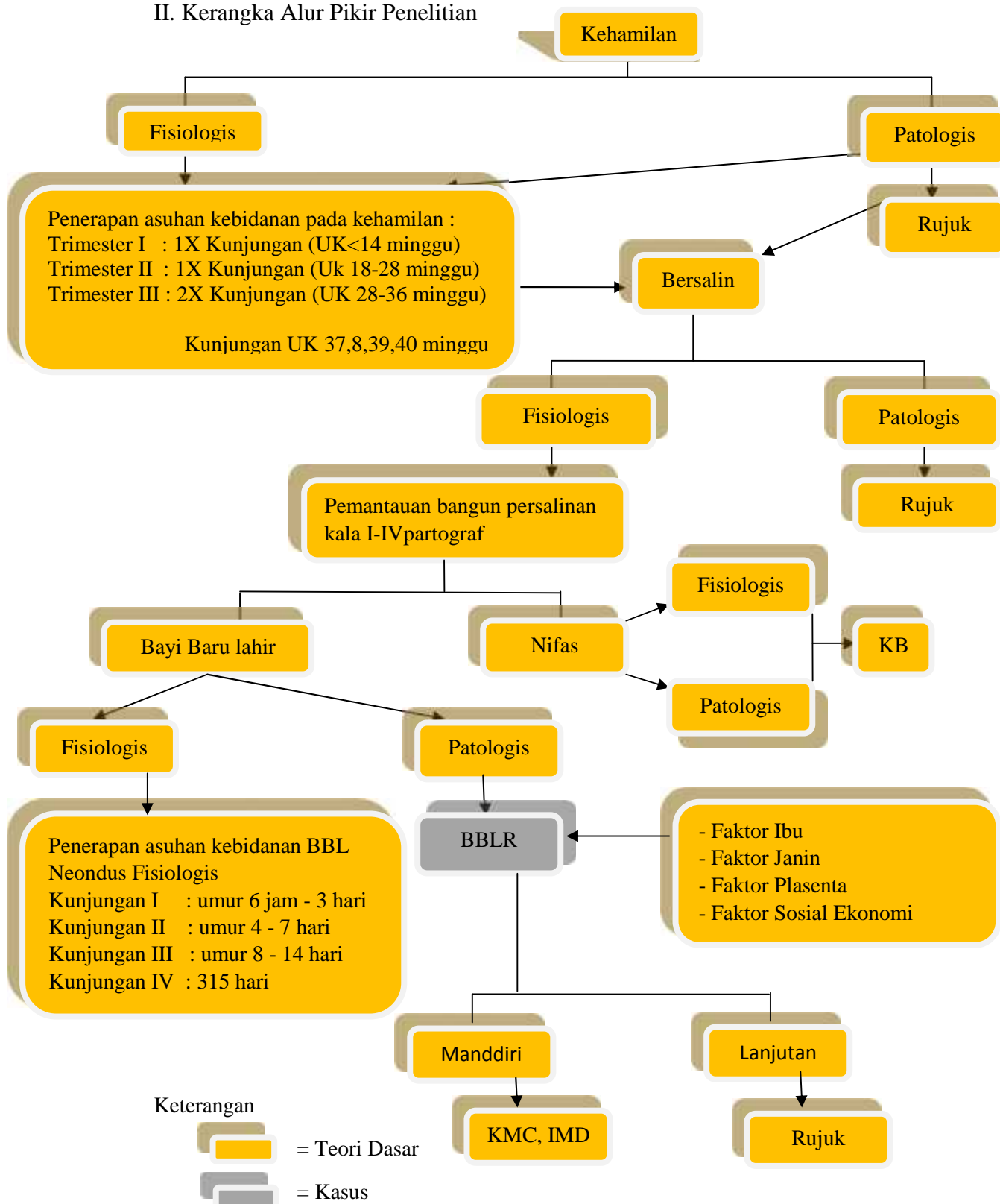
Gambar 2.20 Kerangka Konsep
