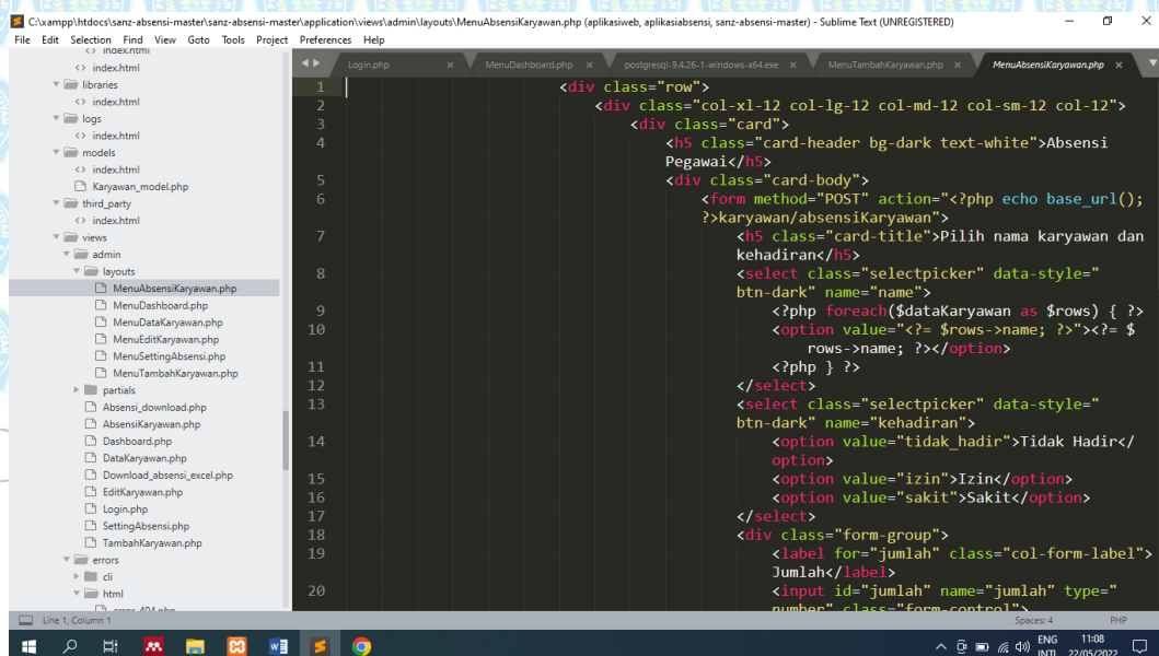
Gambar Data karyawan 4.2.6
